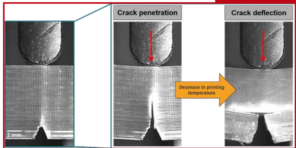
Möglichkeiten der Rissausbreitung. Possibilities of crack propagation.
